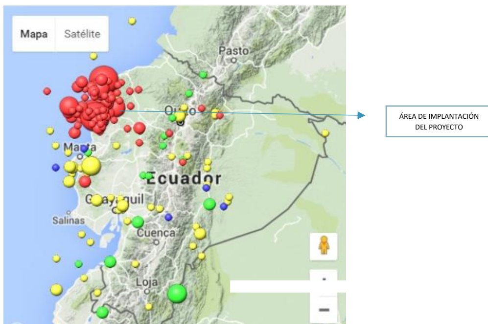
Mapa 4. Terremotos en Ecuador. Fuente: Google Map
