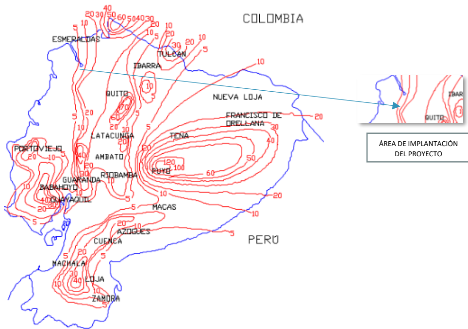
Mapa 11. Amenaza de tormentas. Fuente: ORBEA. E, 2017.
