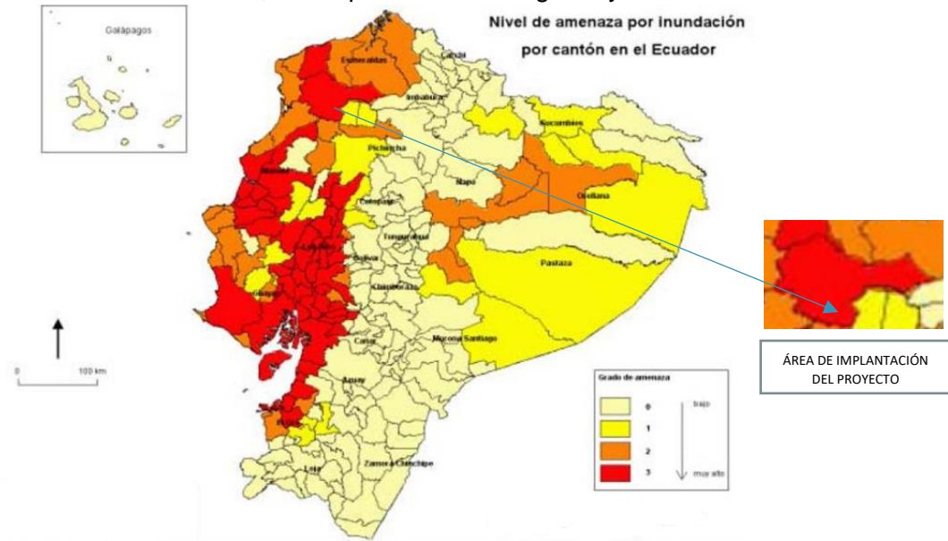
Mapa 9. Amenaza de inundaciones en Ecuador Fuente: IG/EPN-Wolf, Yturralde, Whympfer et al., 2000
