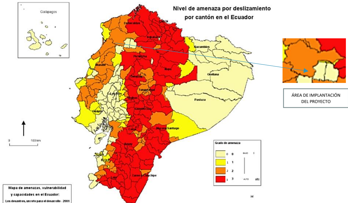
Mapa 6. Amenazas por deslizamiento en Ecuador. Fuente: INAMHI/INFOPLAN- Mapas topográficos del IFM.
