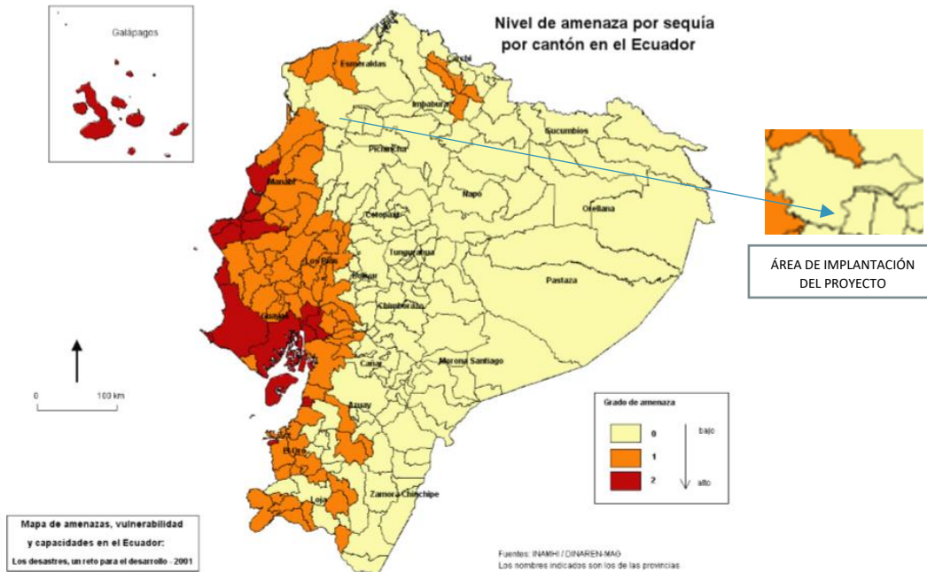
Mapa 10. Amenaza por sequía Fuente: INHAMI/ DINAREN-MAG
