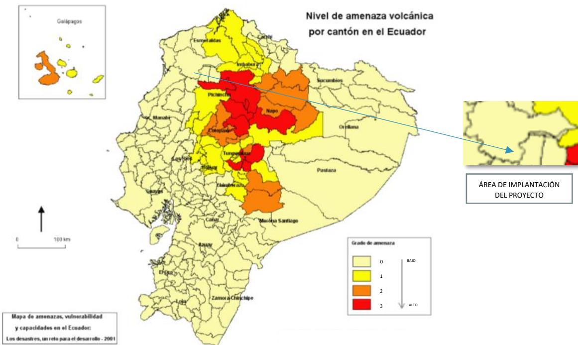
Mapa 7. Amenaza volcánica en Ecuador. Fuente: IG/EPN-Wolf, Yturralde, Whympfer et al., 2000
