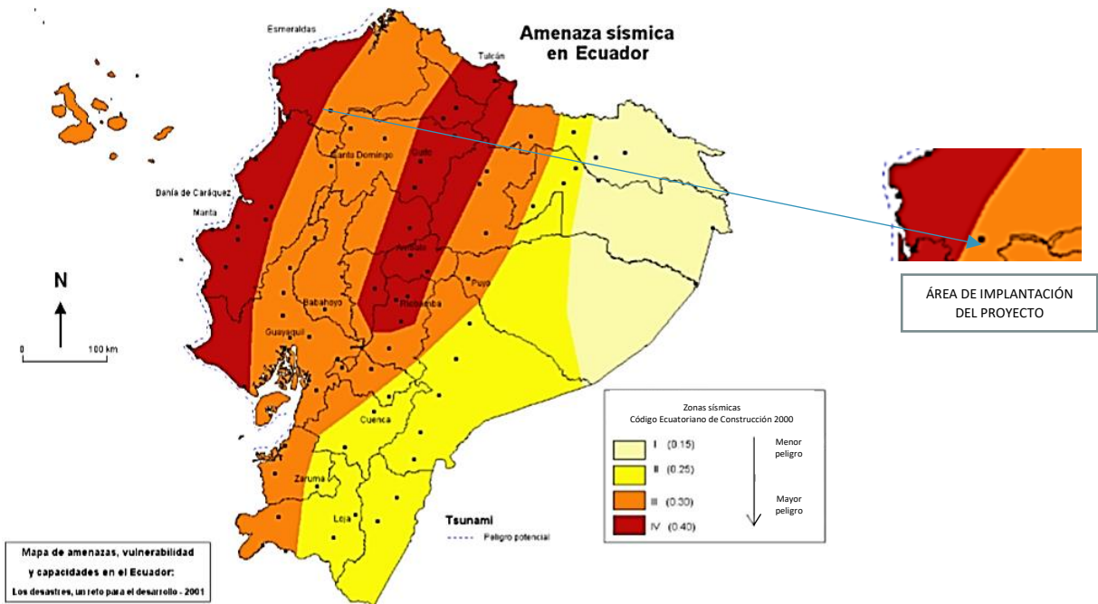
Mapa 5. Riesgo Sísmico en el Ecuador. Fuente: IG/EPN-Wolf, Yturralde, Whympet et al., 2000
