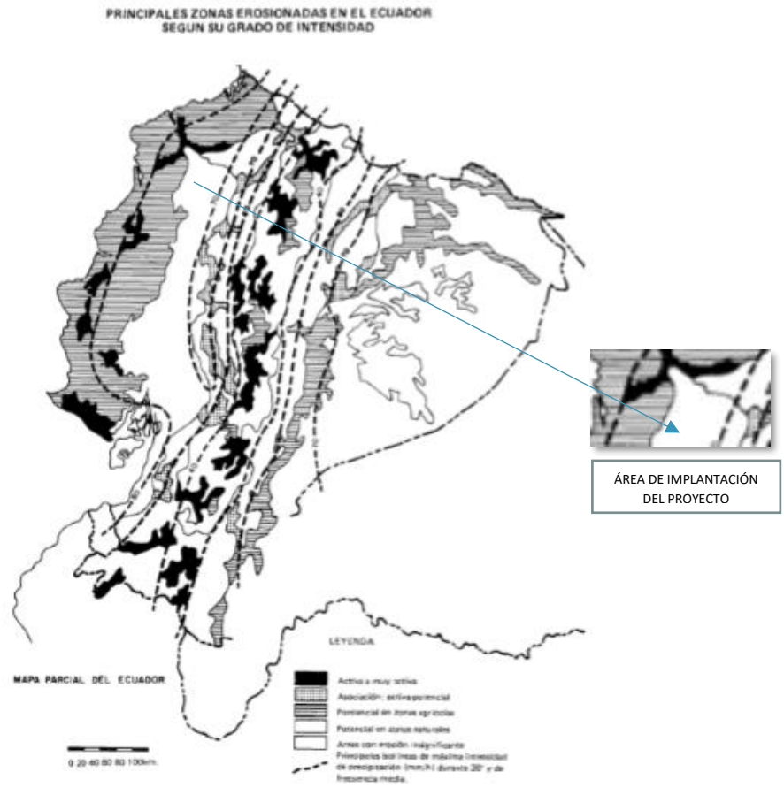
Mapa 8. Erosión en el Ecuador. Fuente: De Noni y Trujillo.
